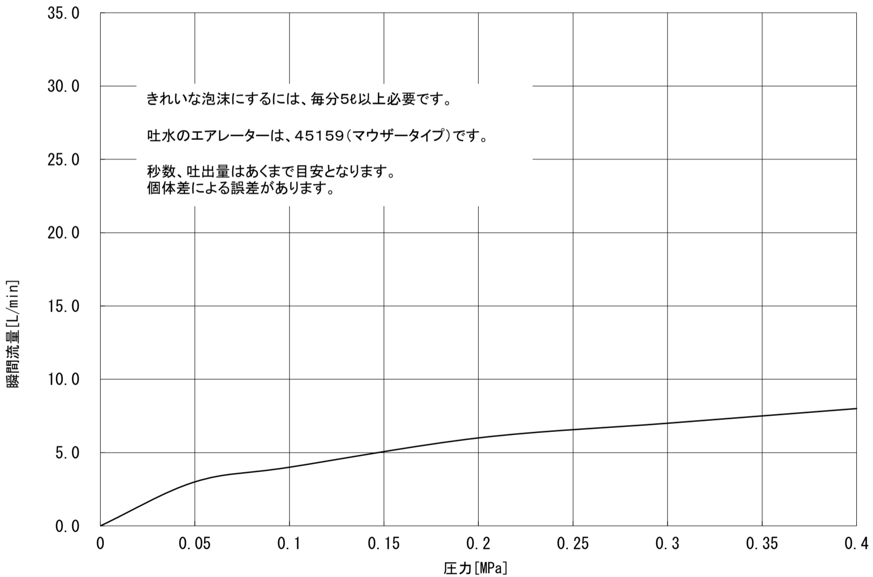
流量曲線
